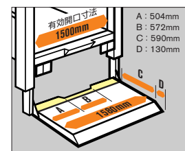
●リフトゲート寸法
