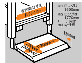
●リフトゲート寸法
